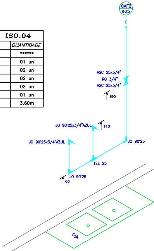
ISOMÉTRICO 04 ESC:..1/25
